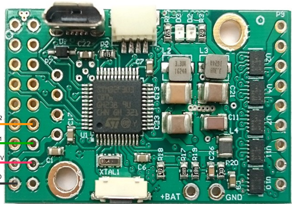
SimpleBGC Tiny rev.B board
